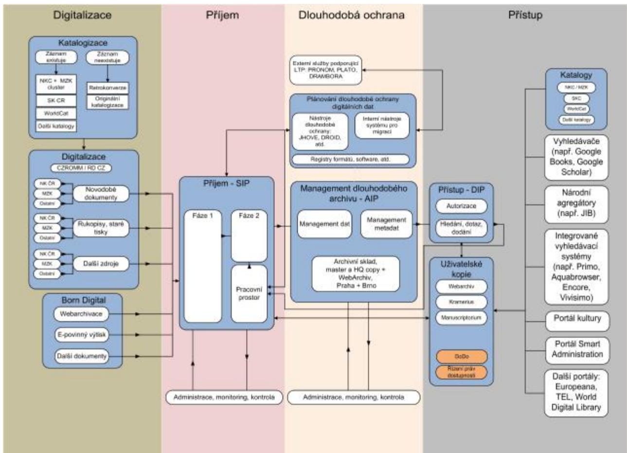
Obr 5: Modifikace modelu OAIS pro workflow NDK
